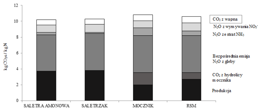
Rys. 5. Ślad węglowy nawozów azotowych z uwzględnieniem CO 2 z wapnowania (produkcja i stosowanie) (na podstawie: Brentrup i in., 2016)
