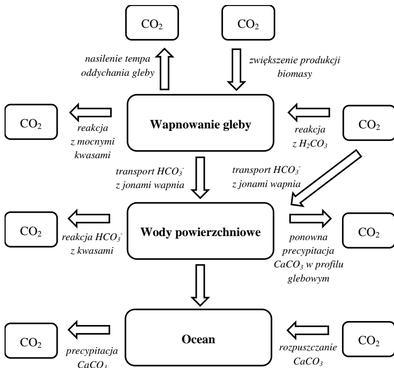
Rys. 4. Przepływ CO 2 po wapnowaniu gleb (na podstawie: Page i in. 2009, Filipek i in. 2015)
