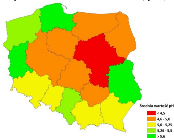
Rys. 1. Przestrzenne zróżnicowanie pH KCl gleb na podstawie statystyk dla województw (źródło danych: Państwowy Monitoring Środowiska – Inspekcja Ochrony Środowiska)
