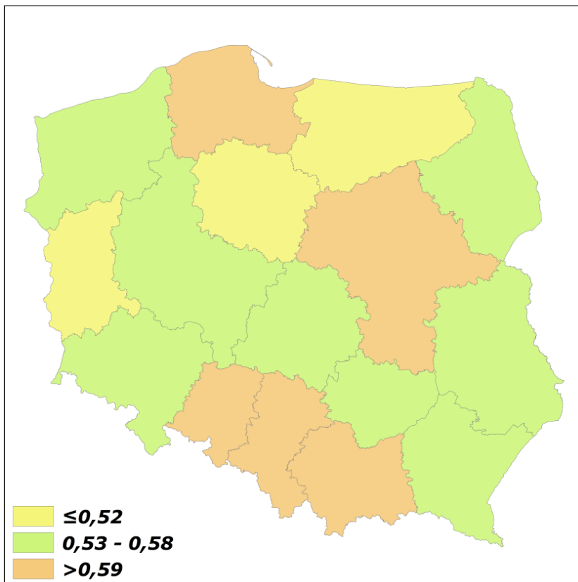
Rys. 5. Grupy województw jednorodnych pod względem sekwestracji węgla organicznego według symulacji DNDC dla uprawy ograniczonej
