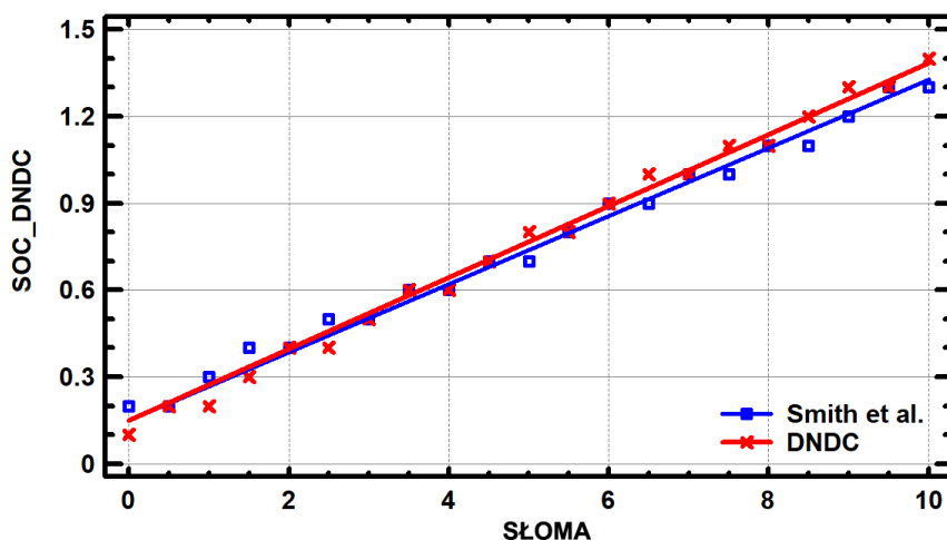
Rys. 3. Przyrosty roczne SOC (%) według DNDC oraz eksperymentalnych meta danych dla Europy w zależności od ilości wprowadzonej do gleby słomy ( t ; wilg. = 15%)
