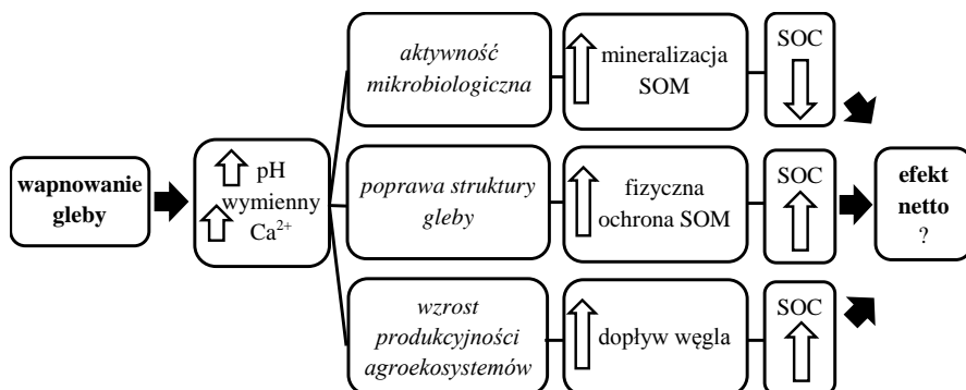
Rys. 6. Potencjalny wpływ wapnowania na zawartość węgla organicznego w glebach (na podstawie: Filipek i in., 2015; Paradelo i in., 2015)
