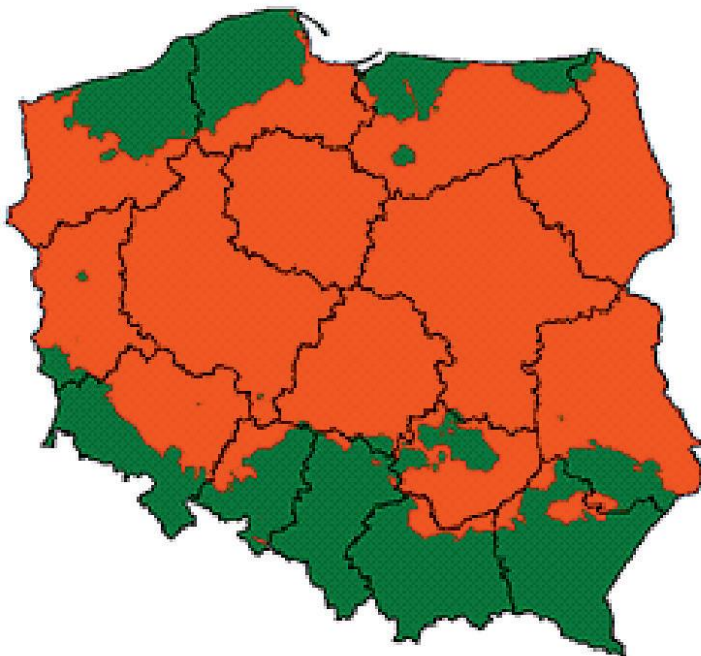
Rys. 1. Regiony klimatyczne Polski według klasyfikacji IPCC (klimat umiarkowany: suchy (kolor czerwony), wilgotny (kolor zielony))
