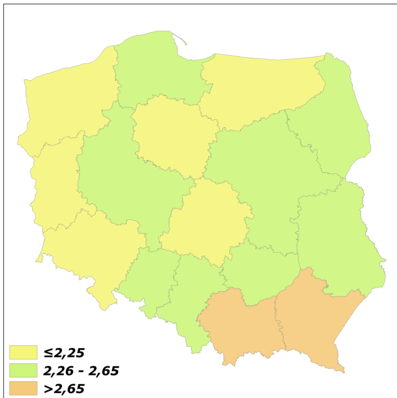
Rys. 6. Grupy województw jednorodnych pod względem sekwestracji węgla organicznego według symulacji DNDC dla siewu bezpośredniego
