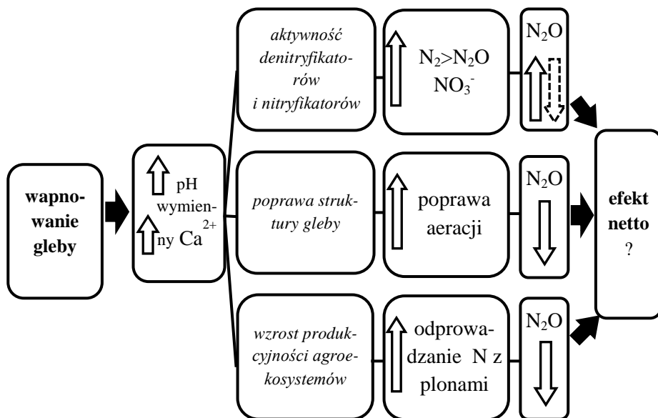
Rys. 7. Potencjalny wpływ wapnowania na emisję N 2 O z gleby
